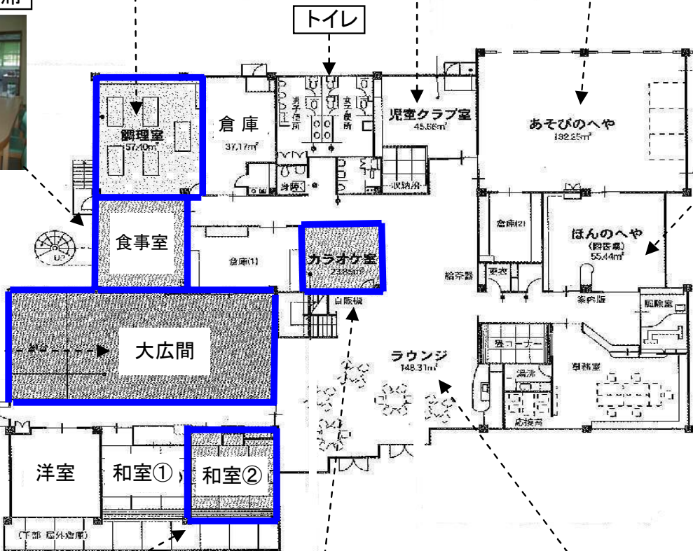
大広間 162.66㎡
