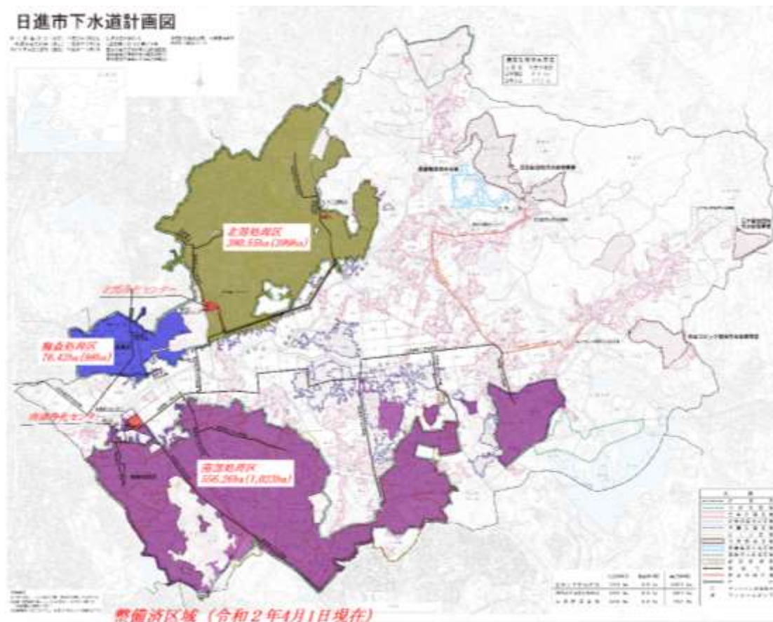
図 公共下水道計画図
